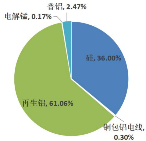
图 6.2“一千克再生铝锭系列产品”的原材料温室气体排放细目
