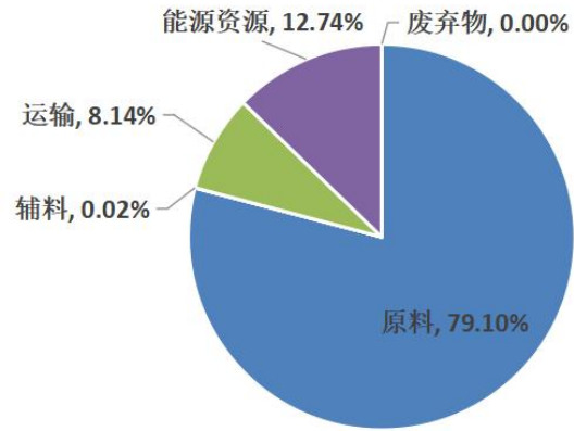
图 6.1“一千克再生铝锭系列产品”的生命周期温室气体排放细目
