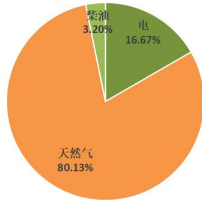
图 6.3 “一千克再生铝锭系列产品”的生产与加工过程能源资源消耗温室气体排放细目
